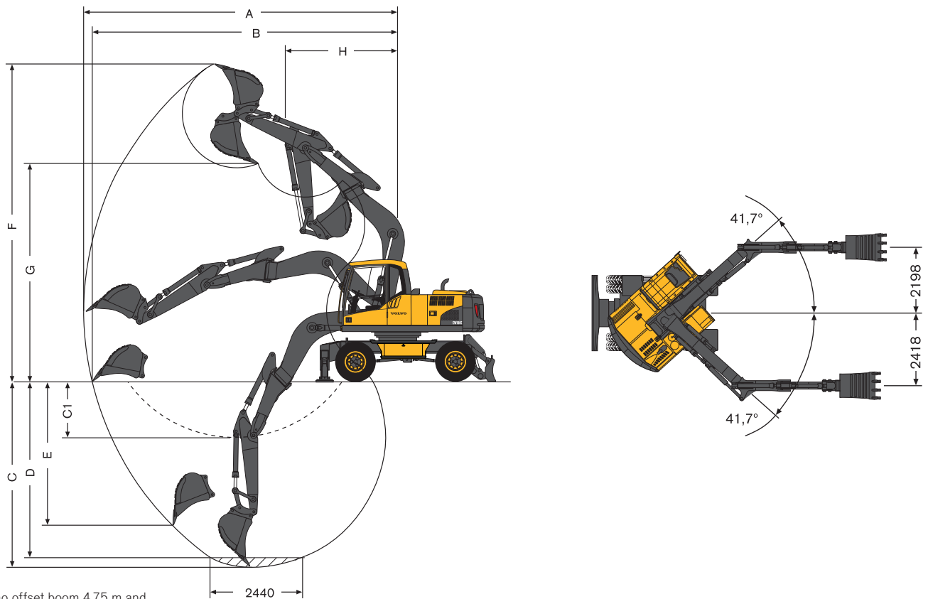
Mono offset boom 4,75 m and dipper arm 2,0 m, 2,45 m, 2,6 m, 3,1 m
