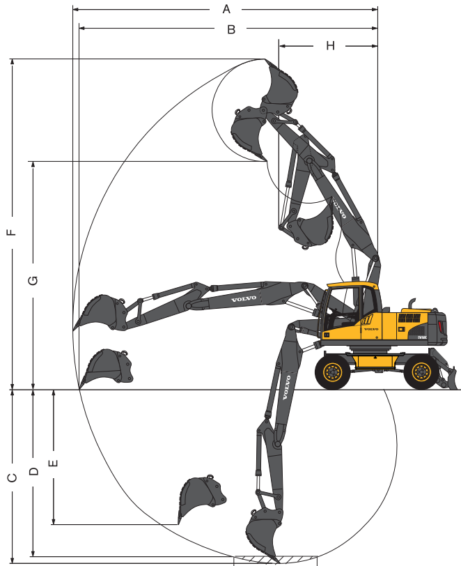
2-piece boom 5,1 m and dipper arm 2,0 m, 2,45 m, 2,6 m, 3,1 m
